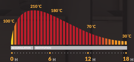
RÉPARTITION DE LA CHALEUR DANS LE TEMPS AVEC LE SYSTÈME DURASIC®
