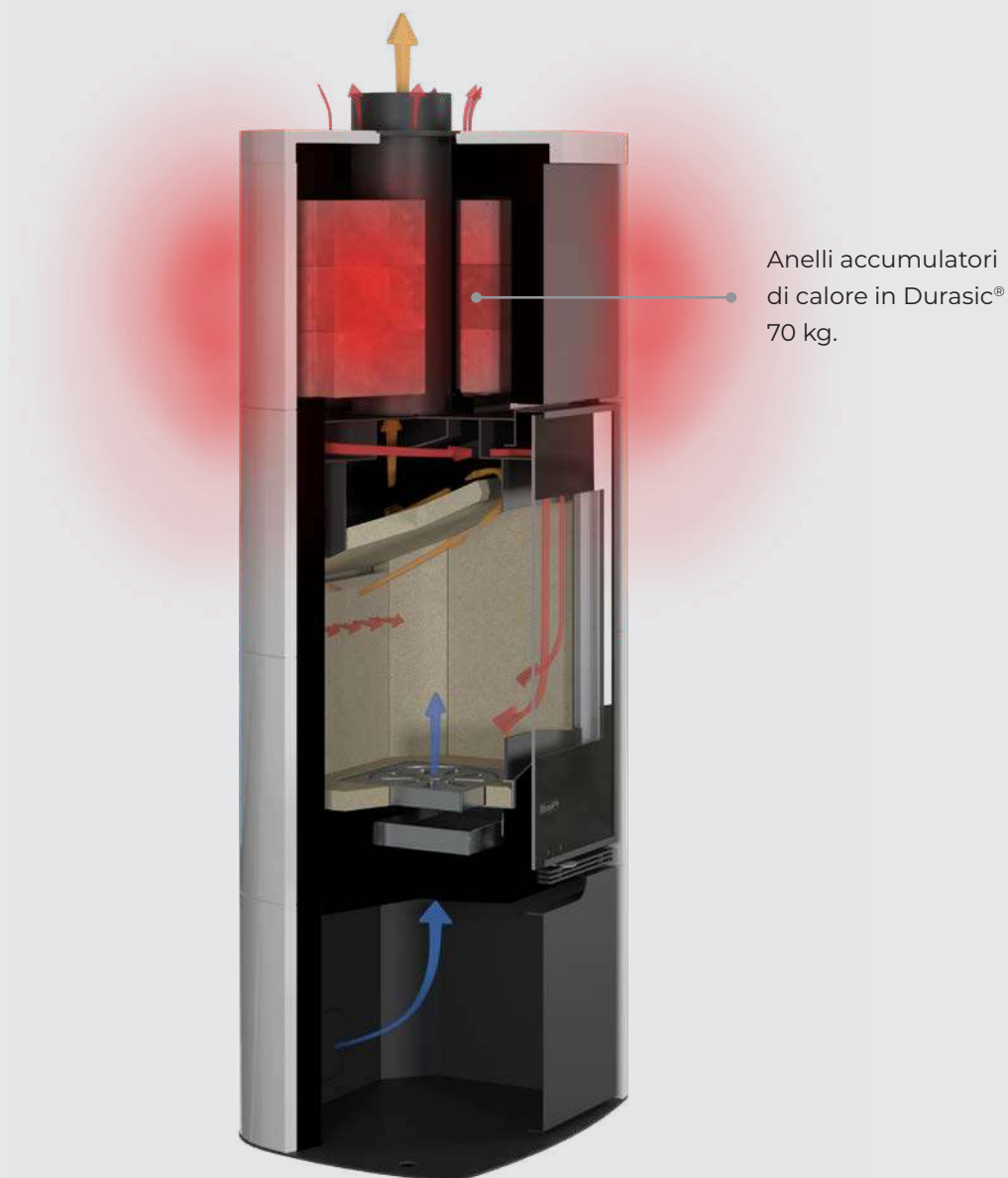
DISTRIBUZIONE DEL CALORE NEL TEMPO CON IL SISTEMA DURASIC®
