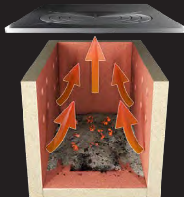
Phase 2: Wärmeabgabe nach der Verbrennung
